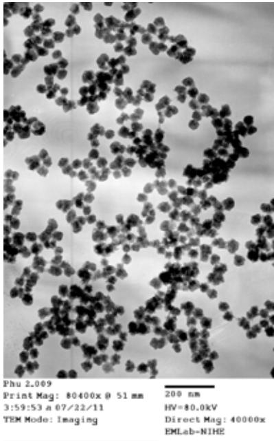
Hình 1: Các hạt nano MnO 2 với độ phóng đại 40000 lần
